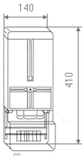
KÖRVONALRAJZ:
