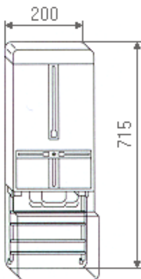
KÖRVONALRAJZ:
