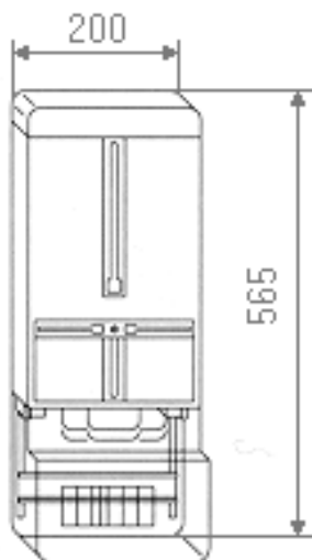
KÖRVONALRAJZ:
